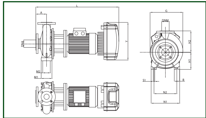
NKM-GE 50-200/219 - NKM-GE 50-250/263
