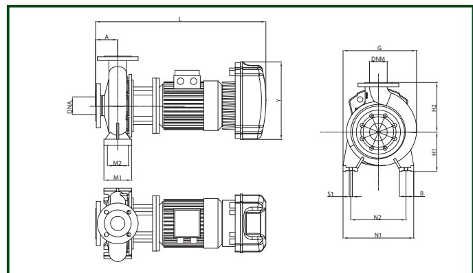
NKM-GE 65-200/219 - NKM-GE 65-250/263
