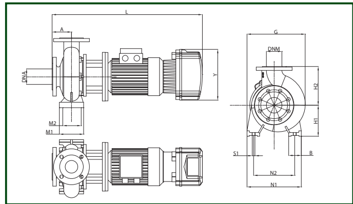
NKM-GE 65-160/177
